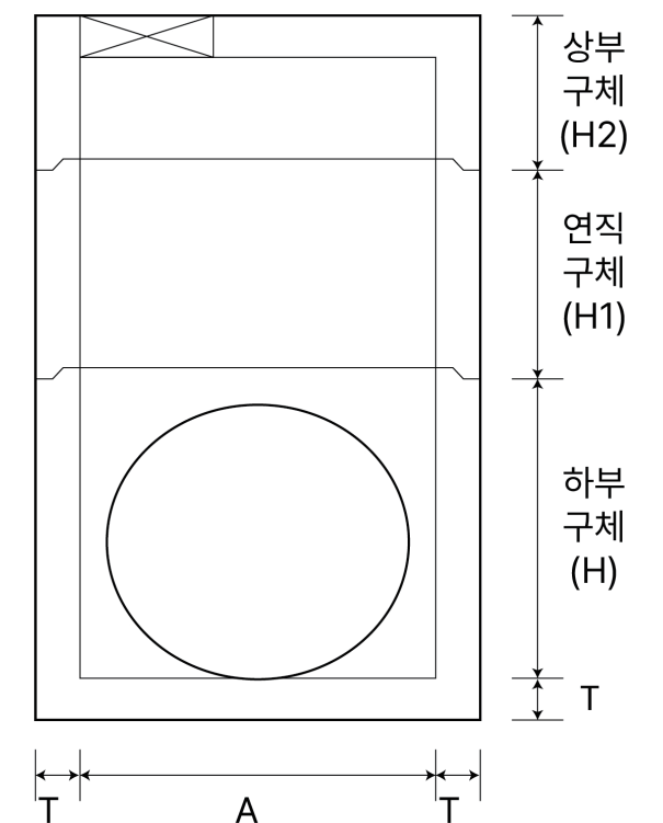
<정면도>
